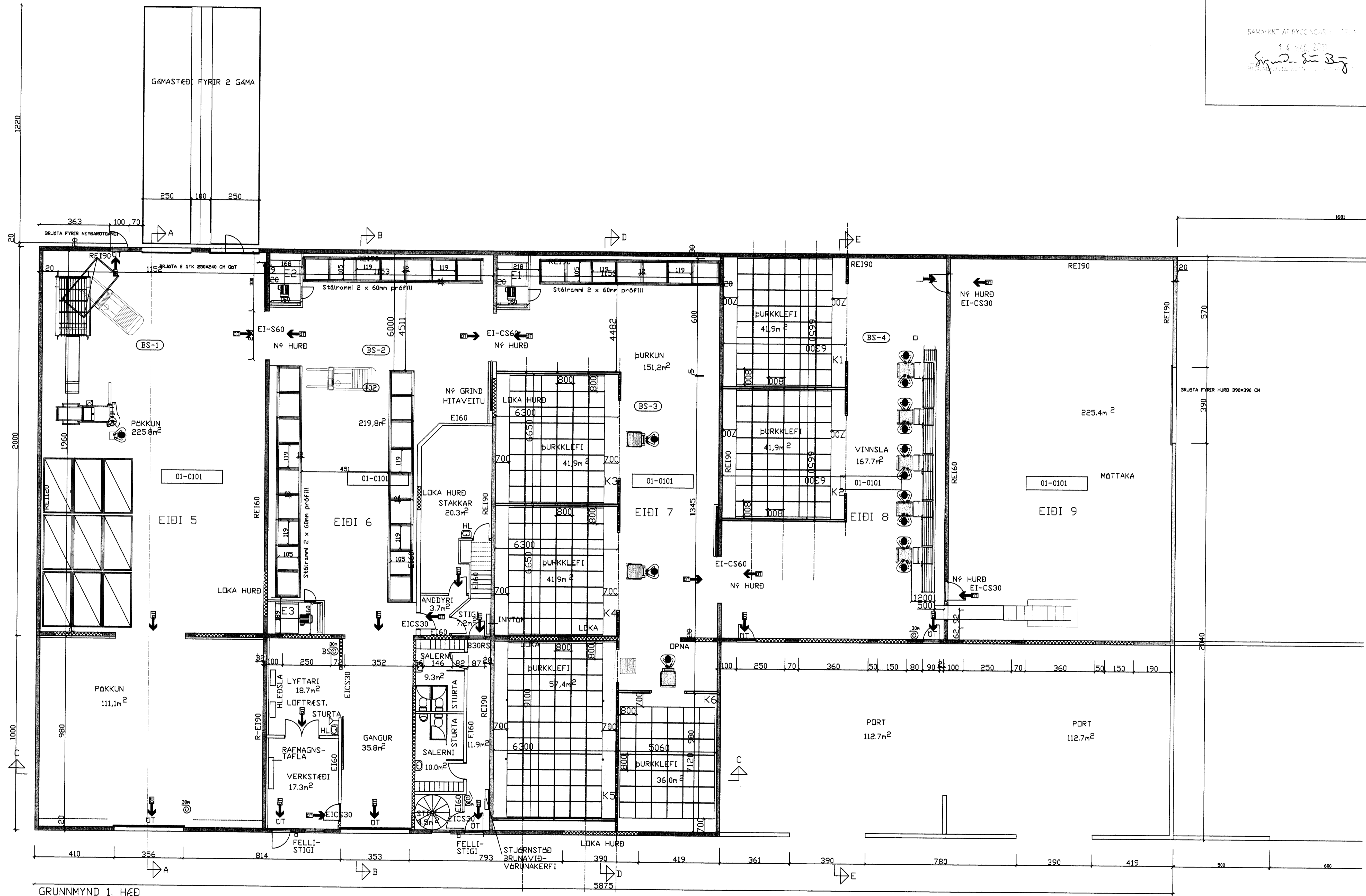
GRUNNMYND 1. HÆÐ
