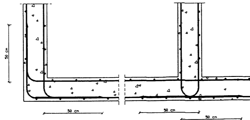
LAGNING LARÉTTRA JÄRNA UM HÖRN Í VEGGJUM M=1:10
