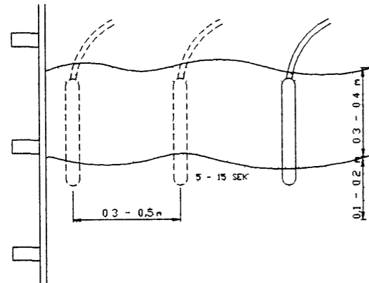
SKYRINGAMYND TITRUM STEYPU Í VEGG
