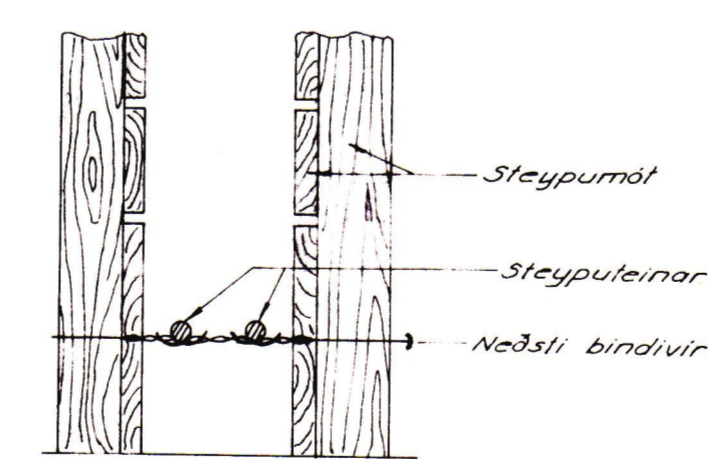
SNID Í SÖKKLI JARDBINDING Í SÖKKLI
