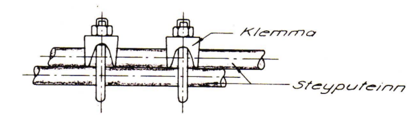
SAMTENGING TRINA ALLAN ÞRINGINN Í SÖKKLINUM
