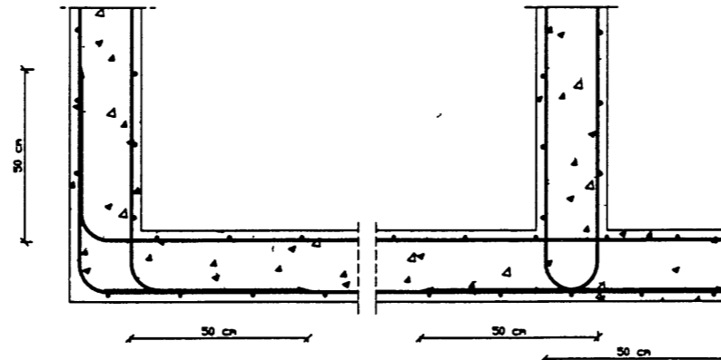
LAGNING LARÉTTRA JARNA UM HÖRN Í VEGGJUM M=1:10
