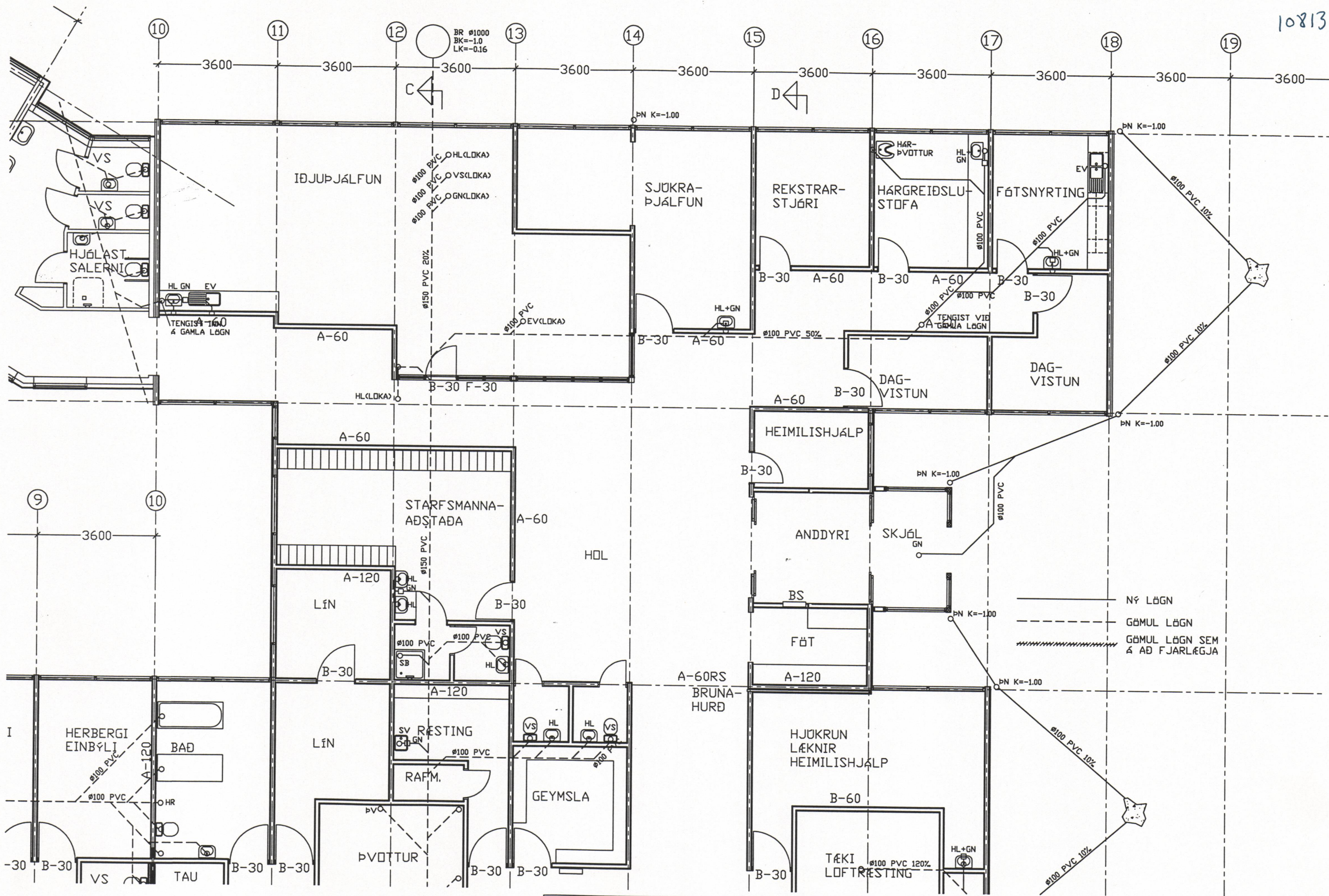
GRUNNMYND NORÐURHLUTI M=1:50
