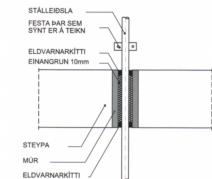
FRÁGANGUR Á STALLEIÐSLU GEGNUM STEYPT GÓLF
