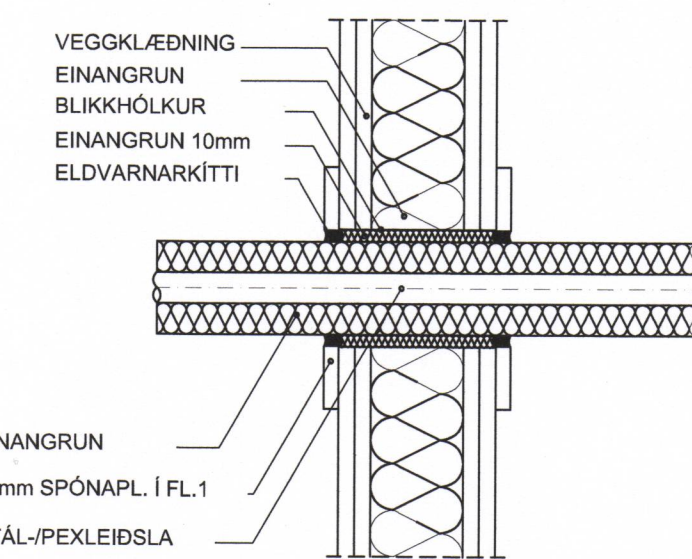
FRÁGANGUR Á STÁL-/PEXLEIÐSLU GEGNUM LÉTTAN VEGG
