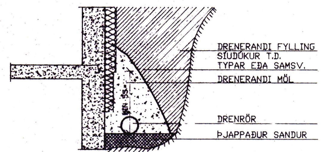
FRÁGANGUR REGNVATNSLAGNAR M=1:20
