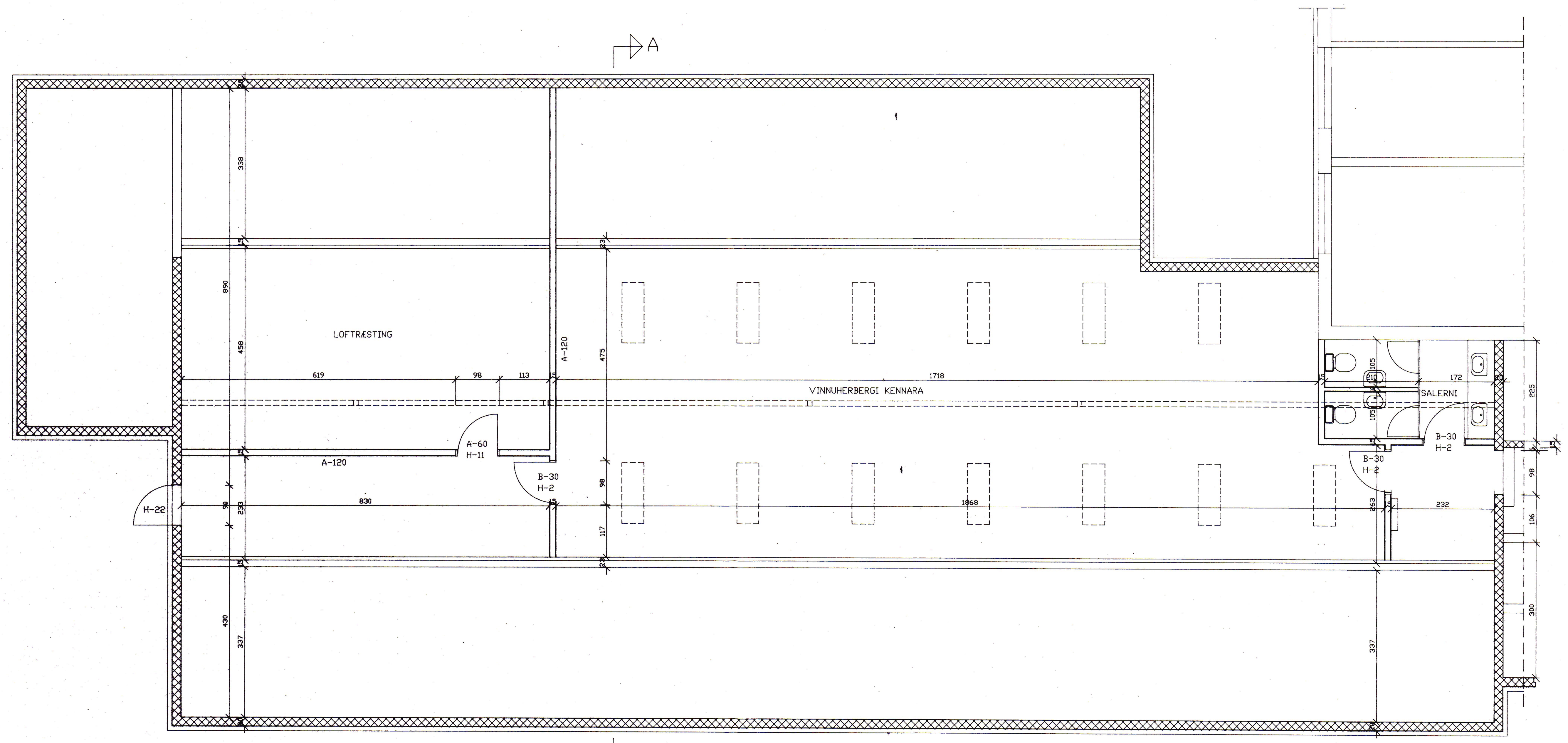
GRUNNMYND 3. HÆÐ M=1:50
