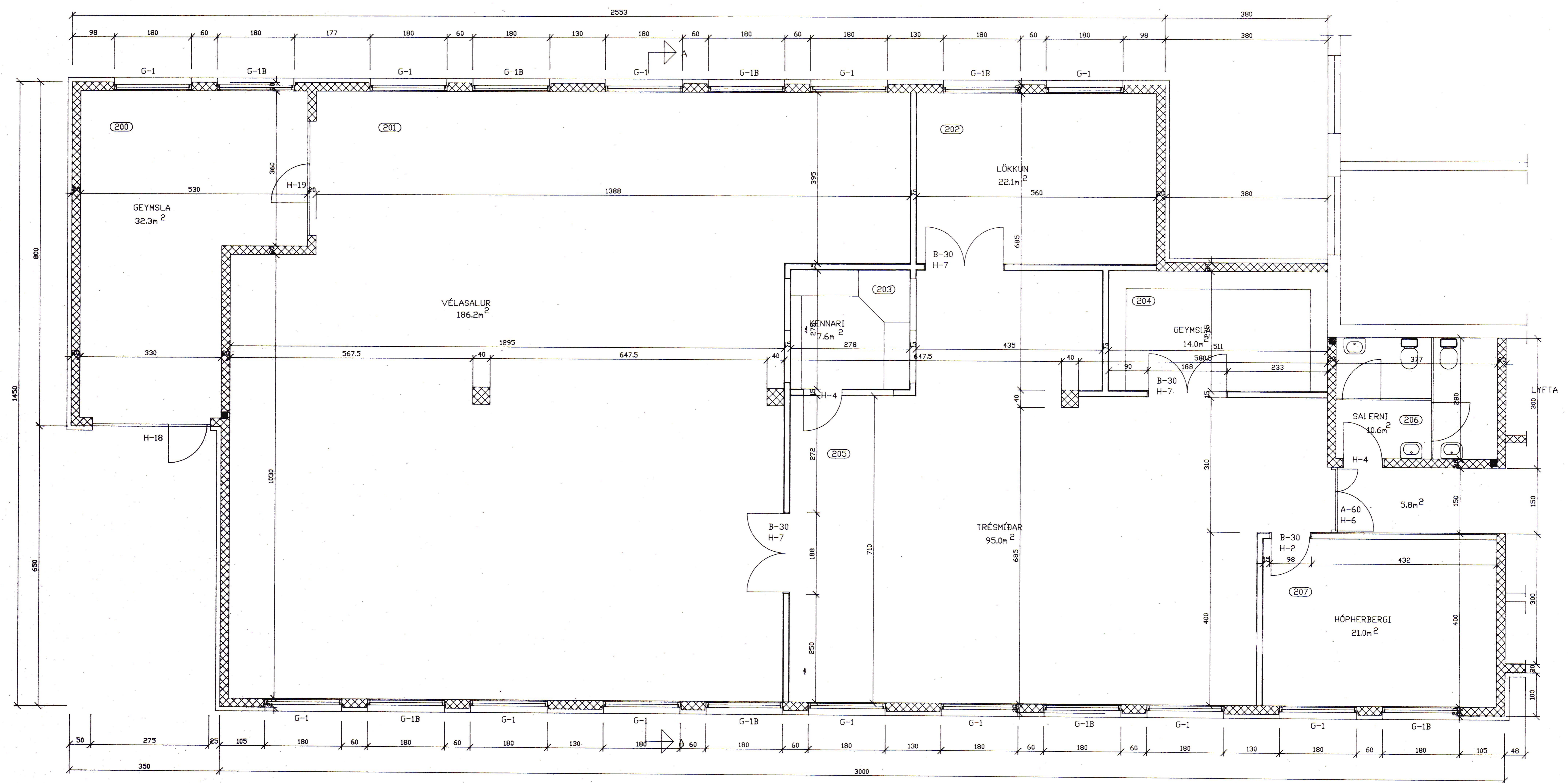
GRUNNMYND 2. HÆÐ M=1:50
