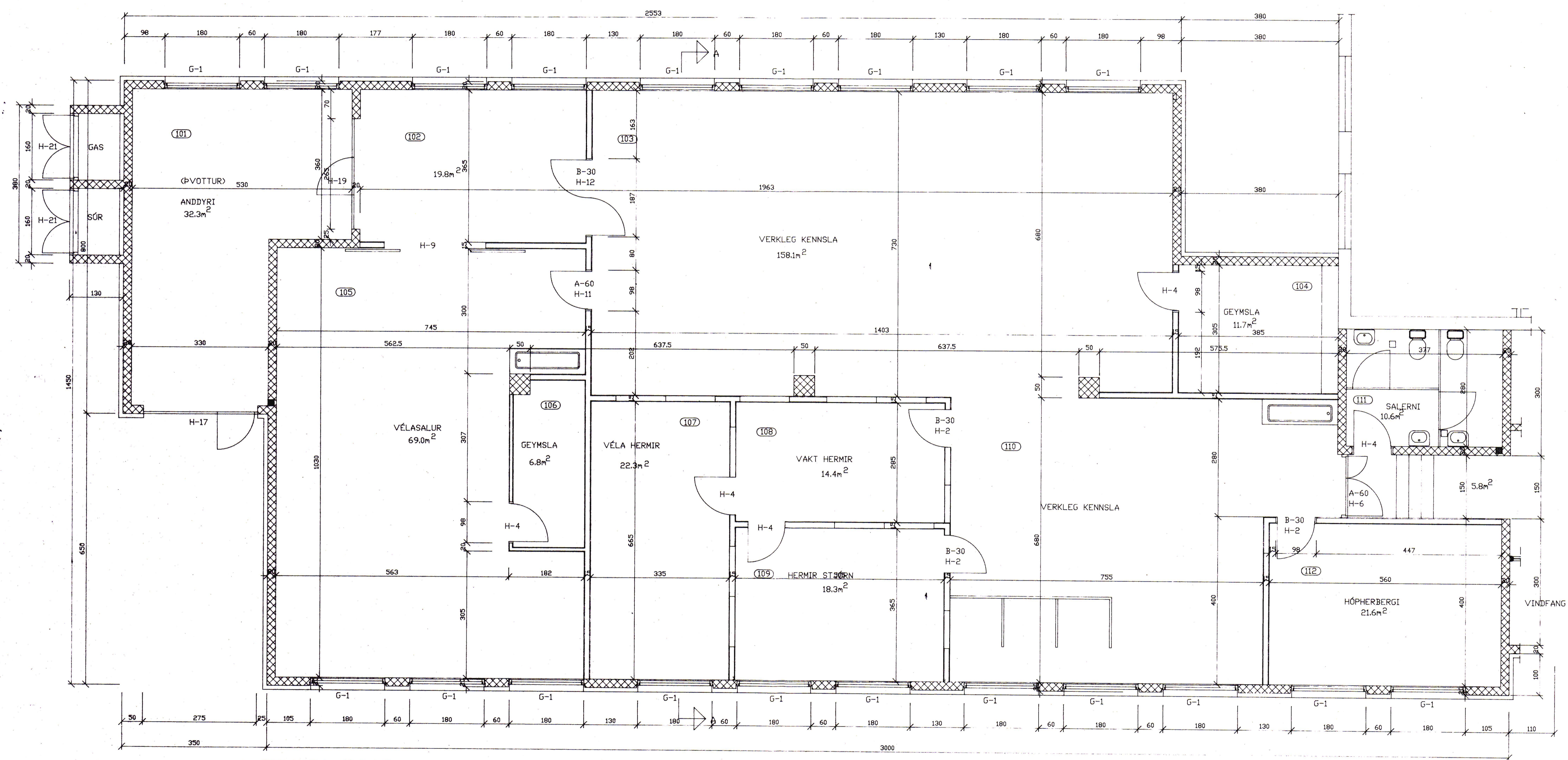
GRUNNMYND 1. HÆÐ M=1:50
