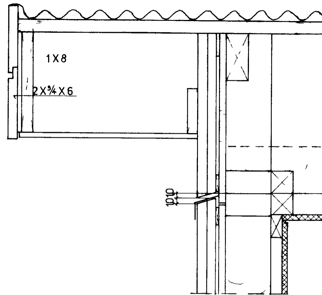
LOÐRETTUR SKURÐUR I STAFN MKV 15
