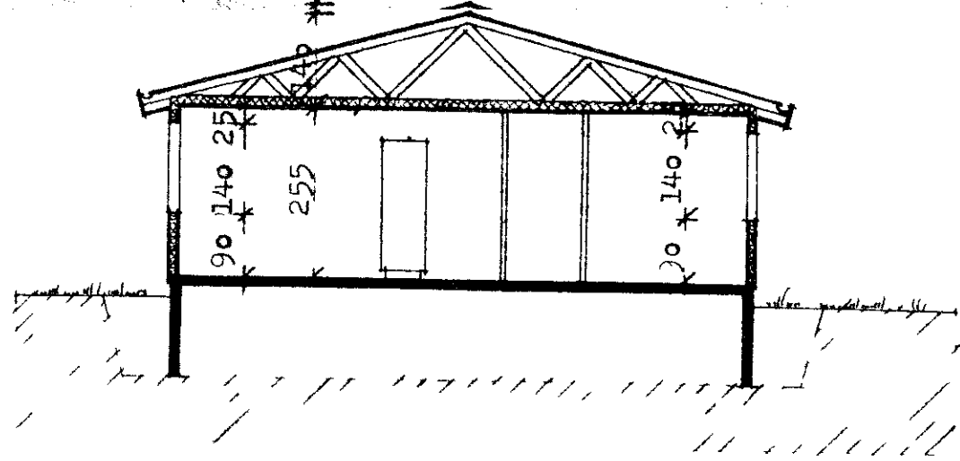
skurður AA
