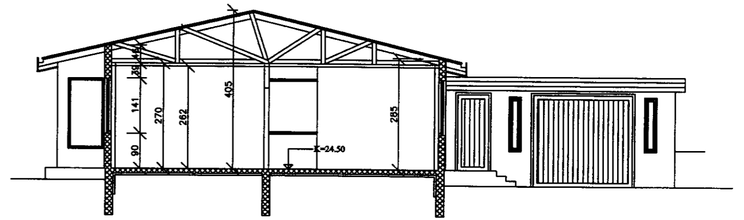
SNIÐ A-A
