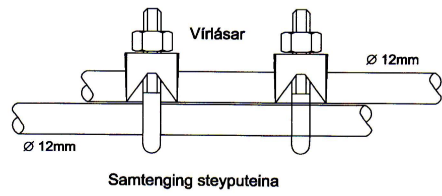
Samtenging steyputeina Setja skal tvo vírlása á hver samskeyti Tengja skal saman tvö neðstu járnin í sökkuleiningum allan úthringinn og að upptaki í tengibox. Í raðhús, parhús og hlíðstæð hús er leiðilegt að tengja sameigilegan úthring en tengibox og tenging verði við hverja heimtaug.
