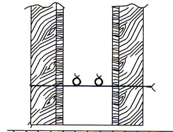
Snið í sökkulvegg Sýnd eru 2 neðstu steypu- styrktarjárn í steypumót ofan á neðstu mótavirum.
