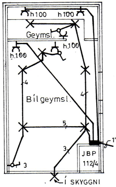
BÍLGEYMSLA 1:100
