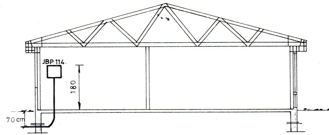
Snið M=1:100
