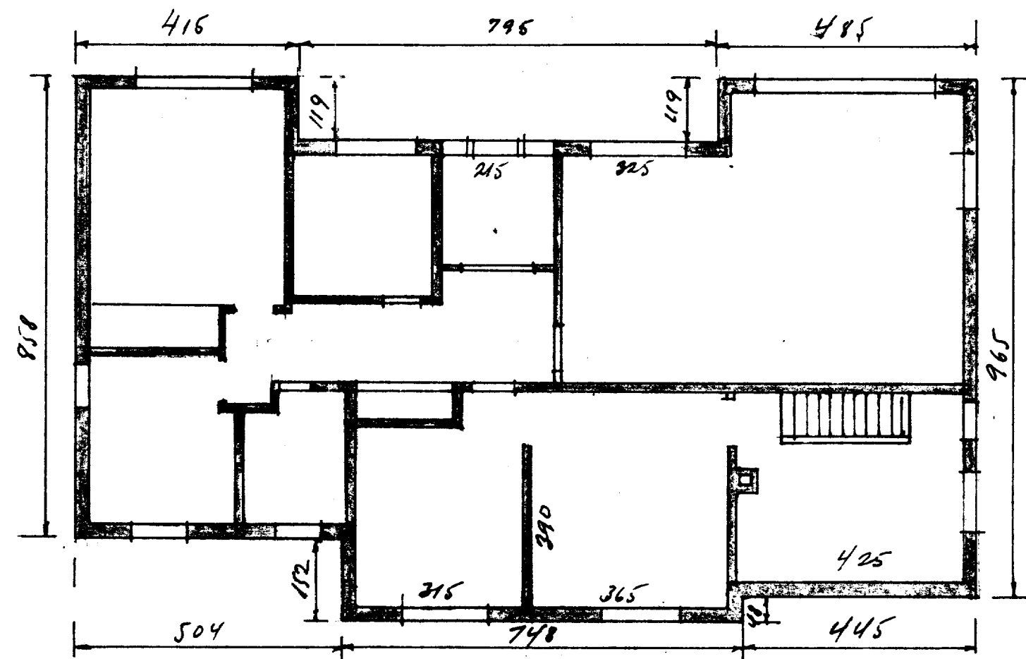
GRUNNFLÖTUR 1. HEB 1:100
