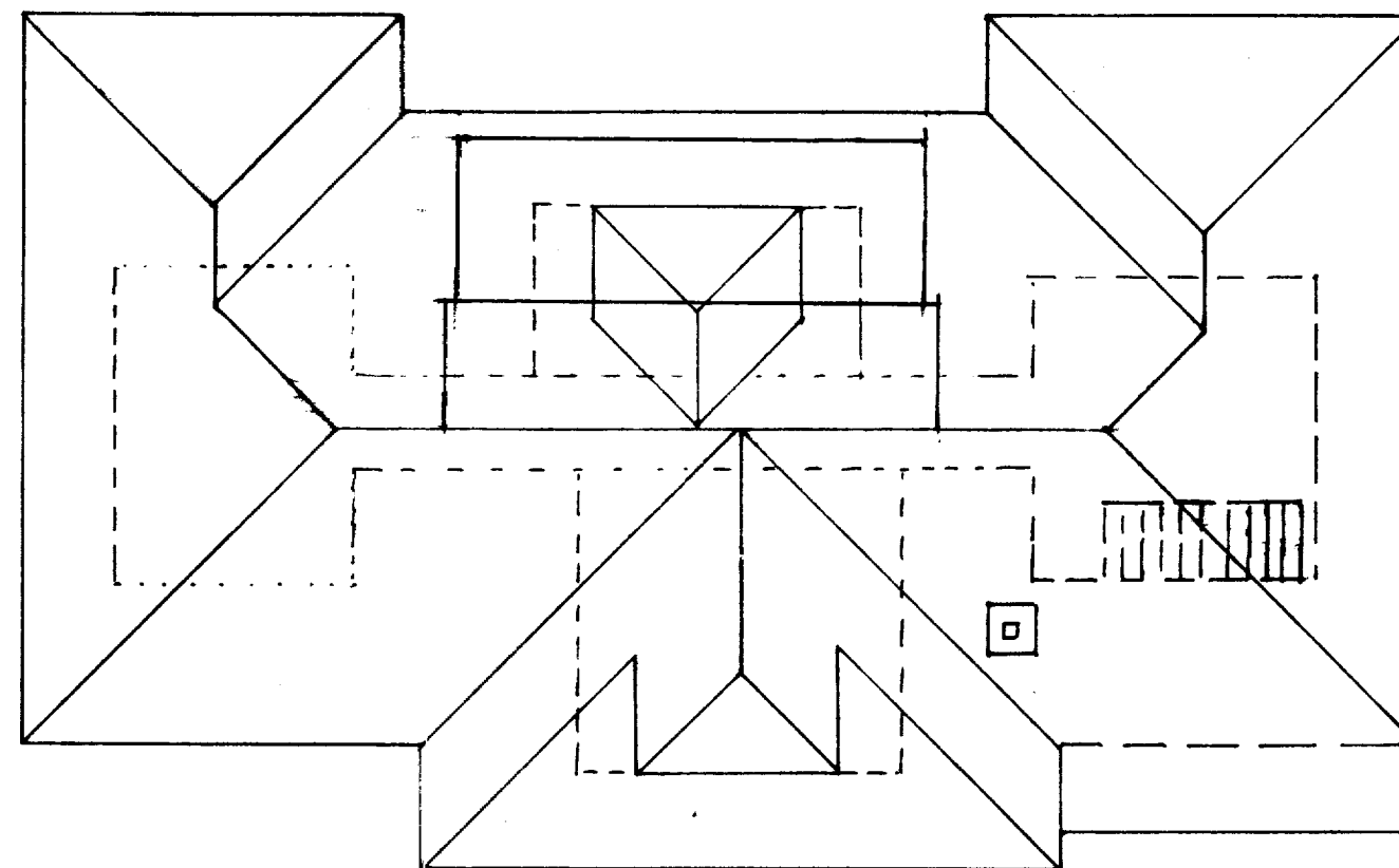
ÞAK
