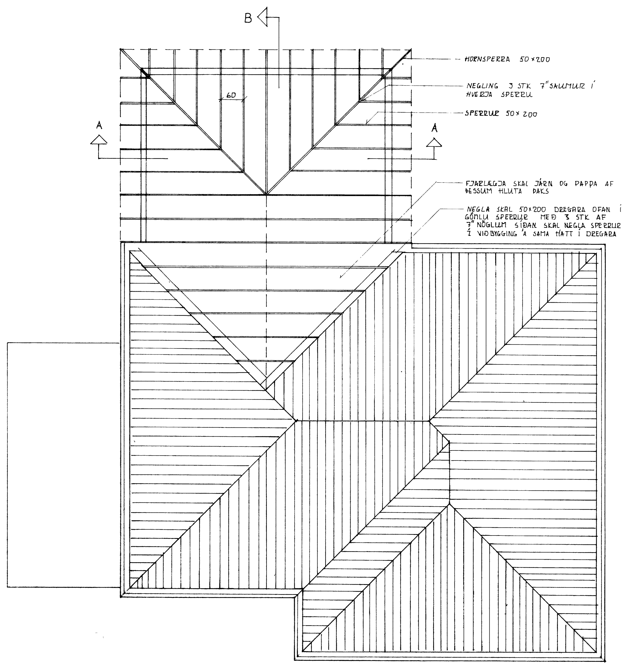
GRUNNMVND ÞAK MKV 1:50
