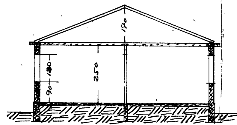
SKURÐUR
