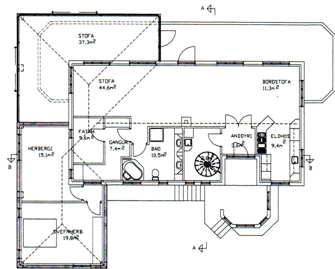
GRUNNMYND 1. HÆÐ
