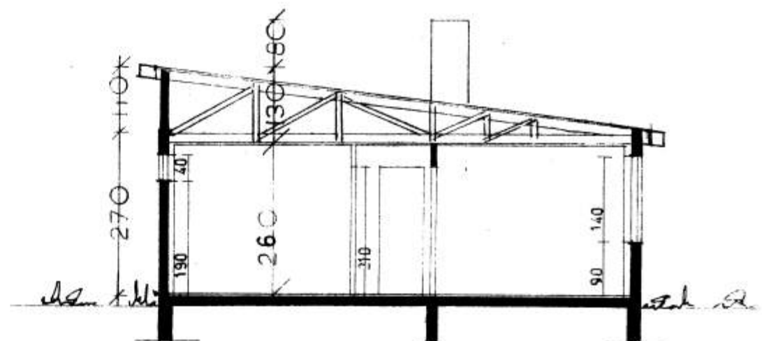
SNEIDING A-A
