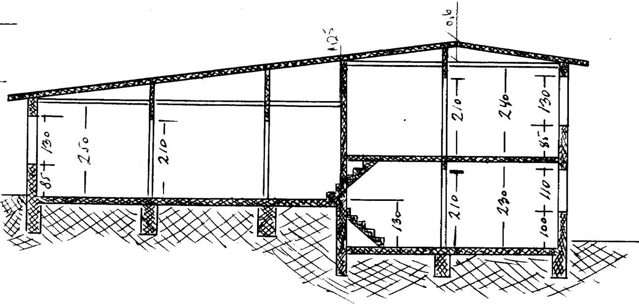
SKURÐUR.
