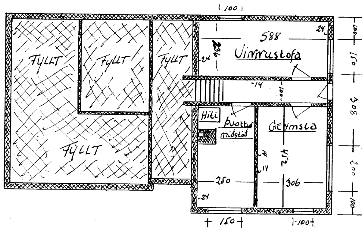
KJALLARI
