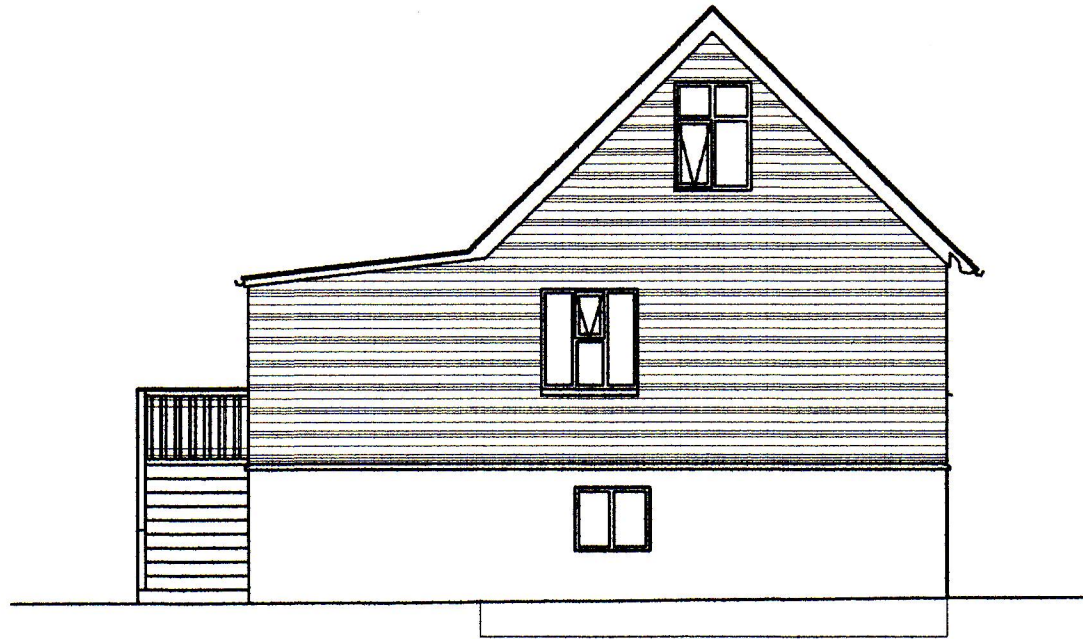
VESTURHLIÐ
