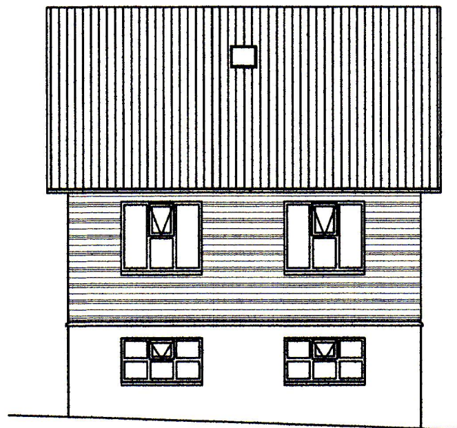
SUÐURHLIÐ
