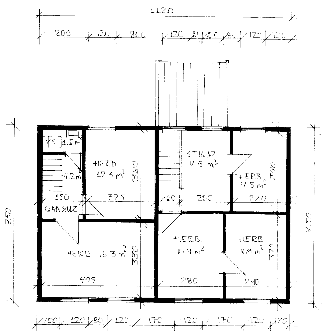
GRUNNMYND 2 HÆÐ MKV 1:100
