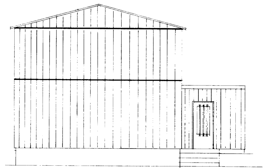
AUSTURHLÍÐ MKV 1:100
