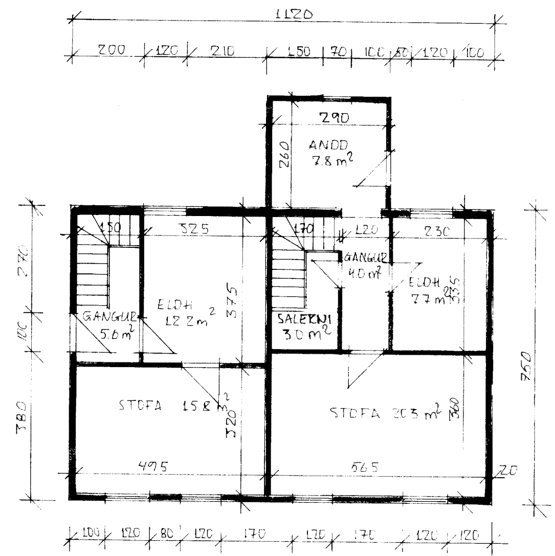
GRUNNMYND 1 HÆÐ MKV 1:100
