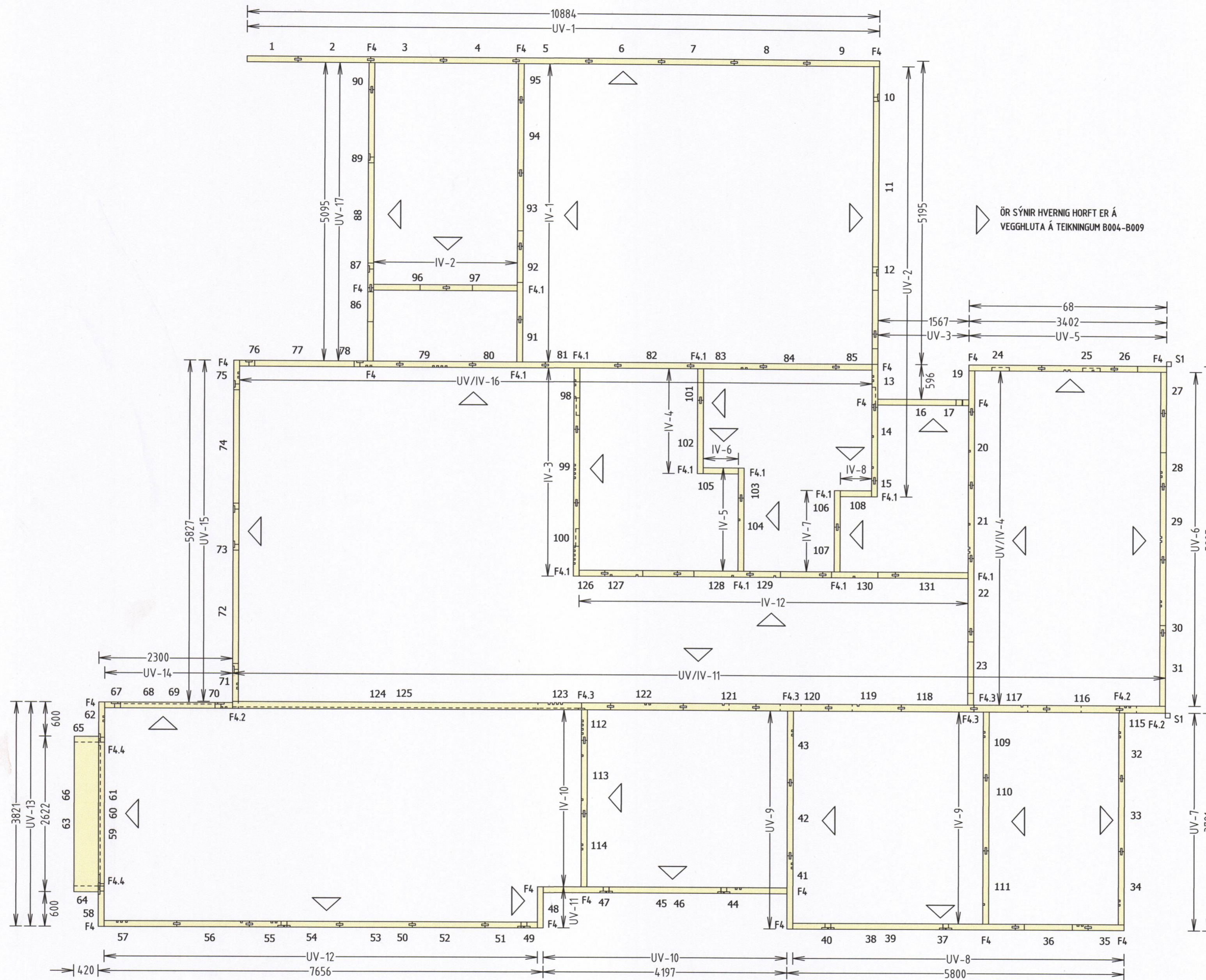
VEGGIR GRUNNMYND 1:50 ÞYKKT VEGGEININGA ÚTVEGGIR 100 mm, INNVEGGIR 100 og 120 mm
