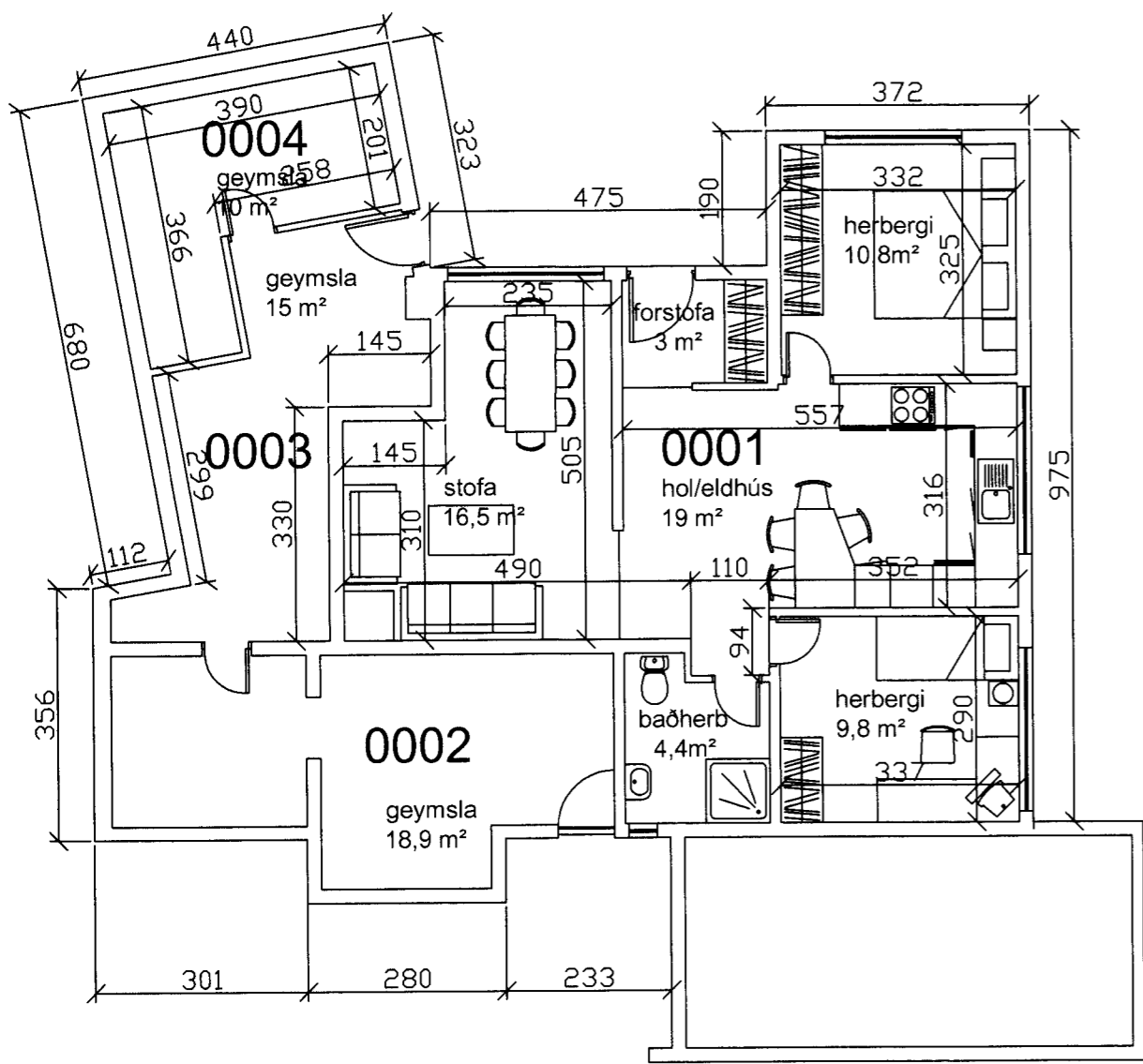
grunnmynd kjallara mkv 1:100
