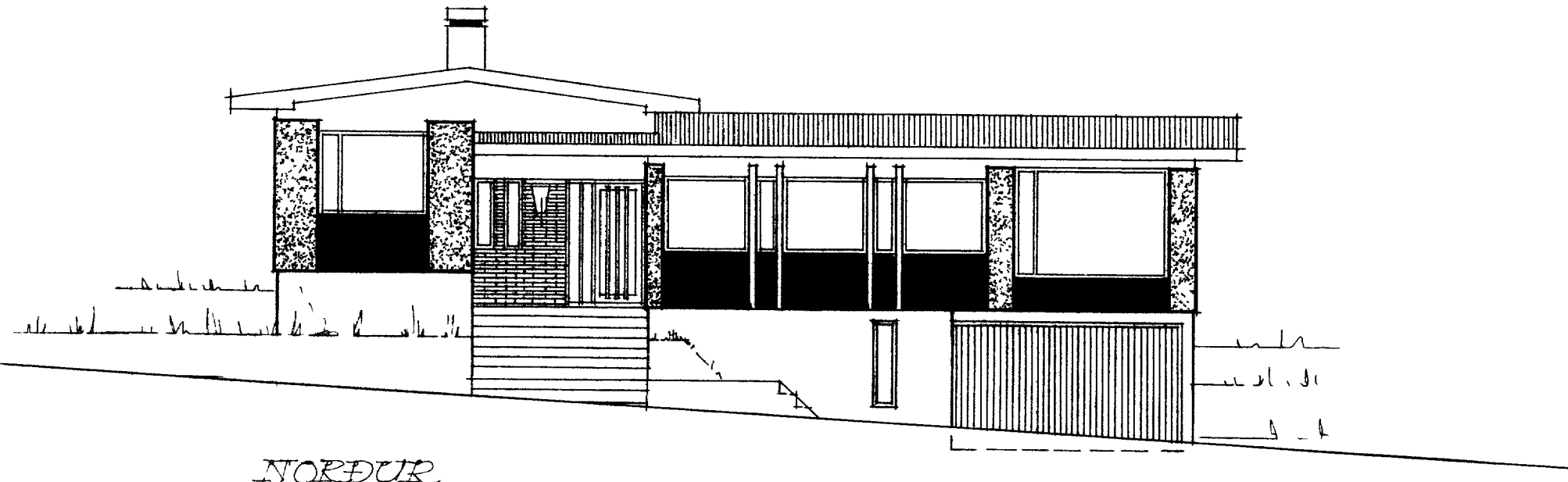
NORÐUR
