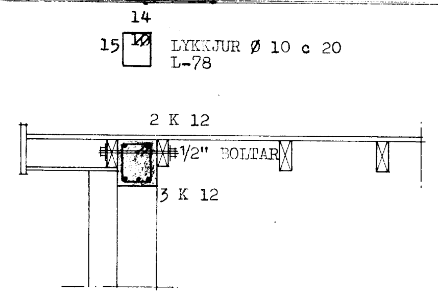
SNID - B 1:20
