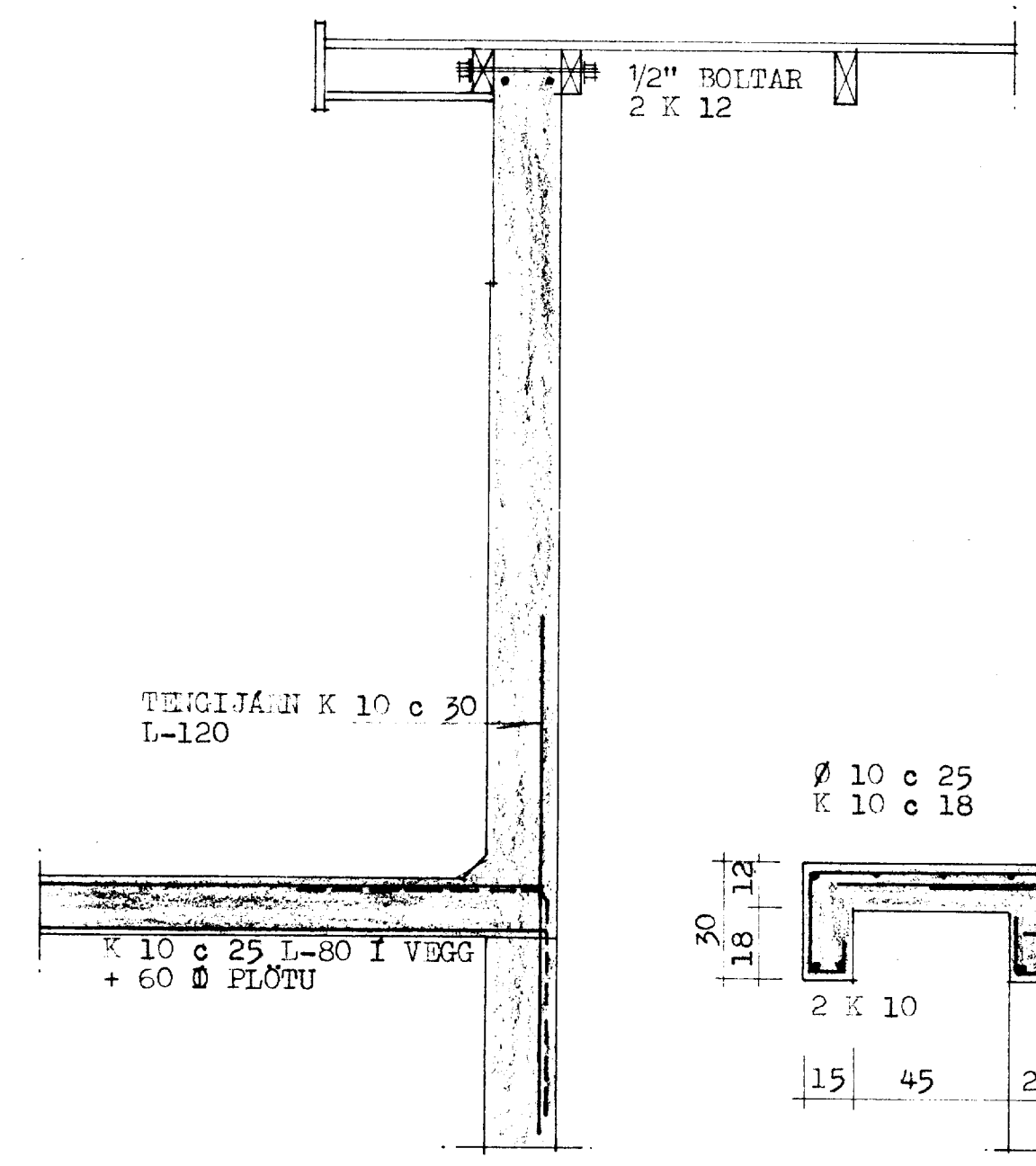
SNID - D 1:20
