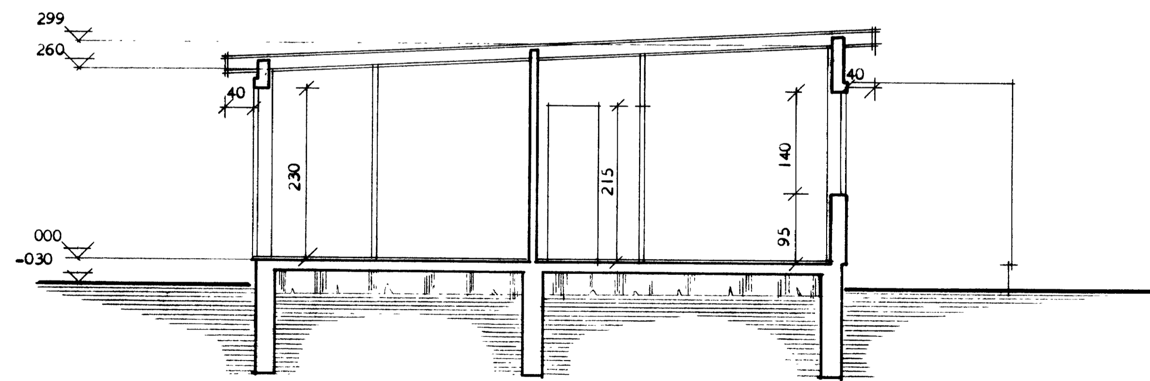
SNEIDING B---B
