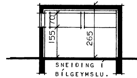
SNEIÐING
