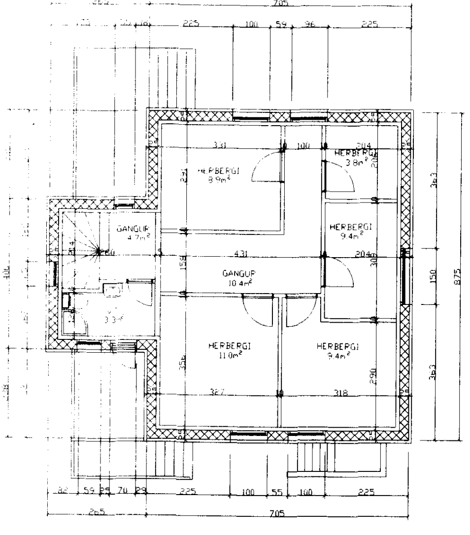
GRUNNMYND 2 HÆÐ M=1:100
