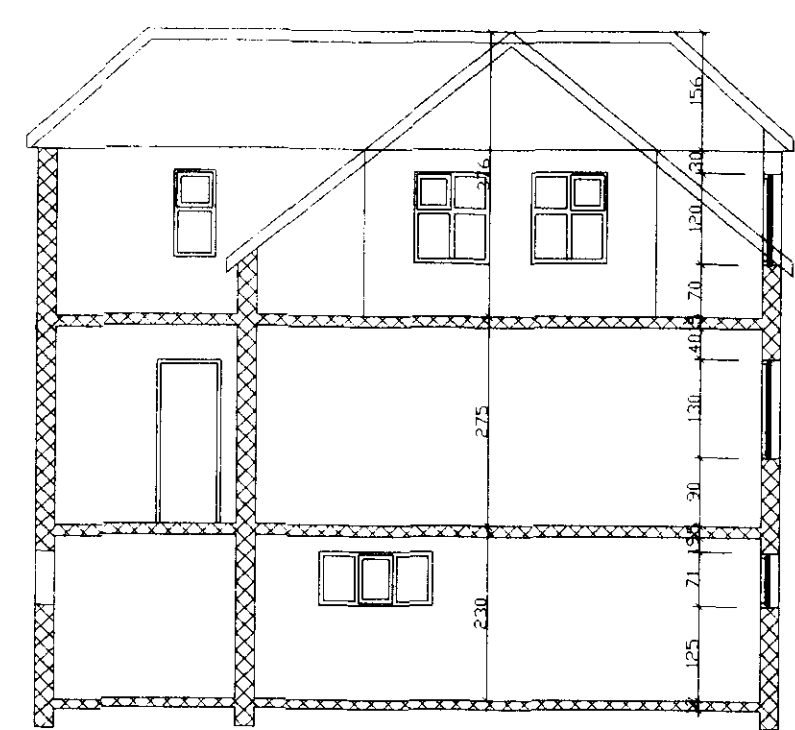
SNIÐ
