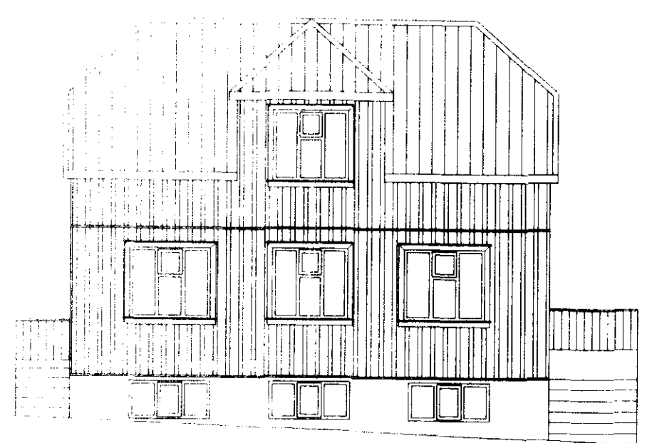
ÁTTIÐURHLÍÐ M=1:100
