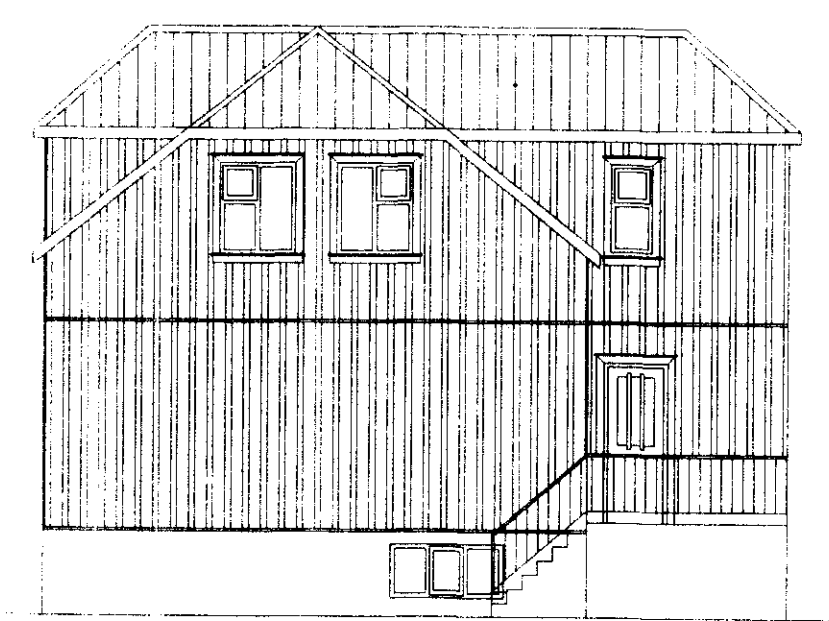
NDRIÐURHLÍÐ M=1:100
