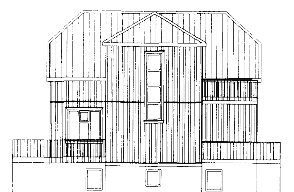
VÆSTURHLÍÐ M=1:100
