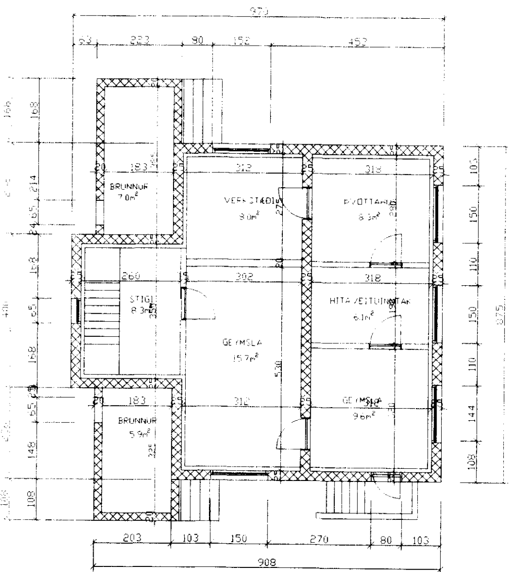
GRUNNMYND KJALLARI HÆÐ M=1:100
