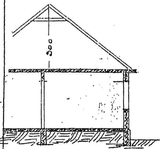
SKURÐUR
