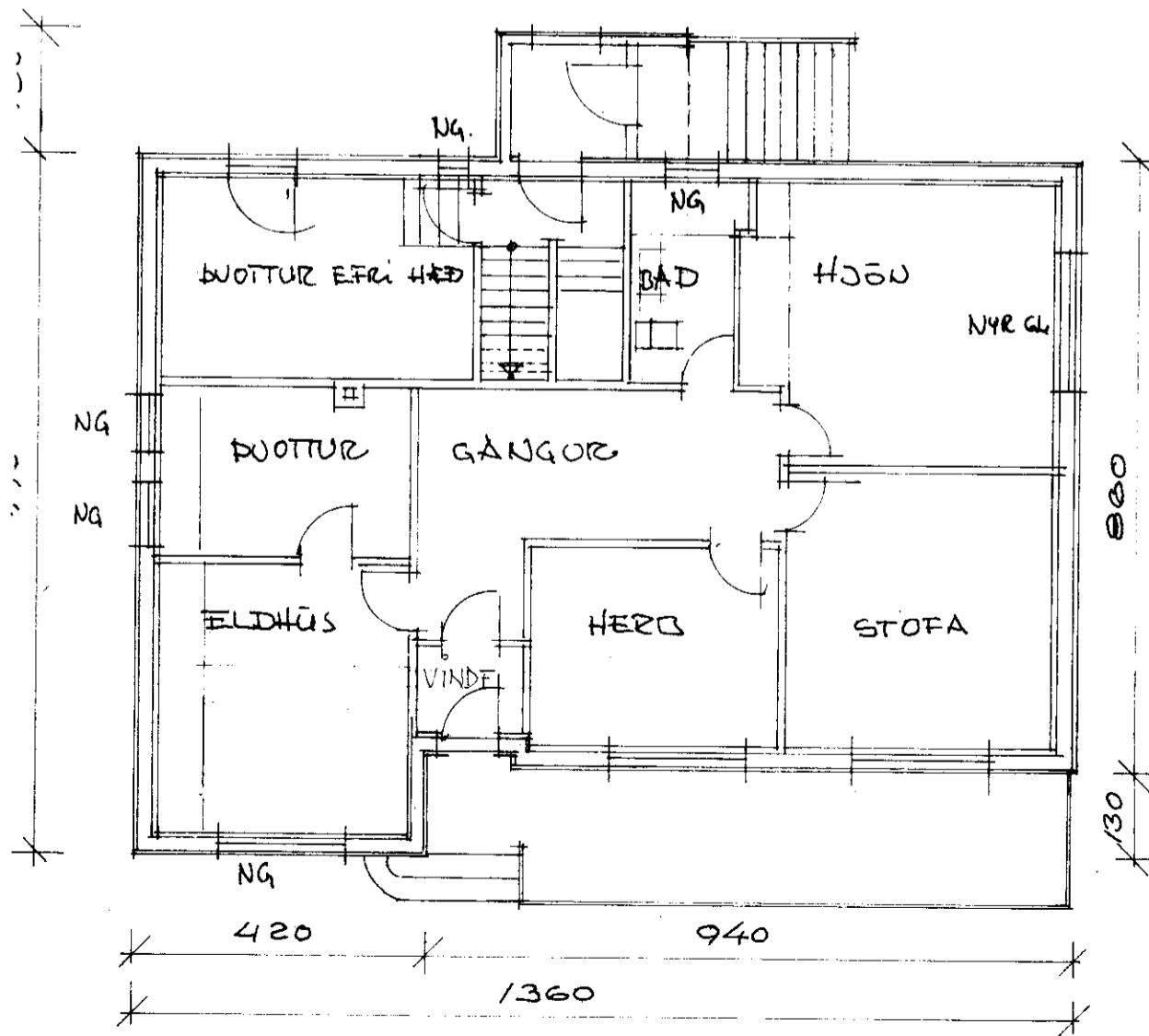
GRUNNMYND 1. HÆÐ 1:100
