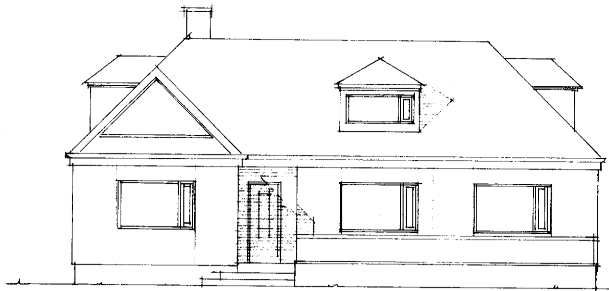
VESTURHLÍÐ
