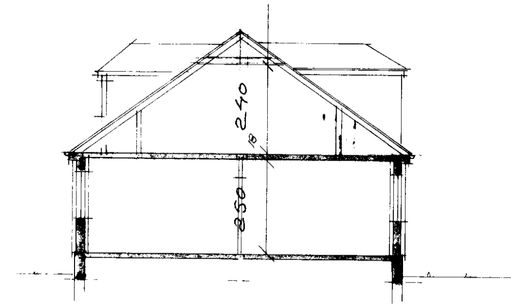
DUERSNIÐ
