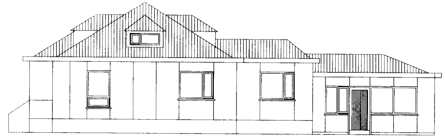
SUDURHLID M=1:100
