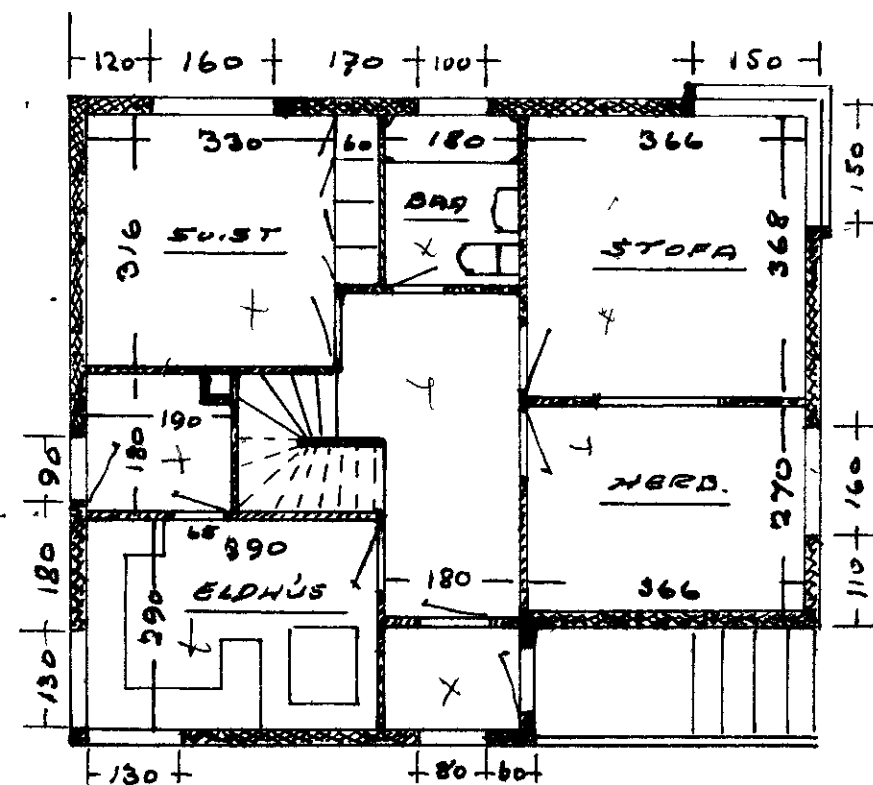
1. HÆÐ
