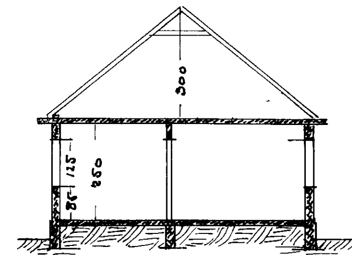
SKURÐUR
