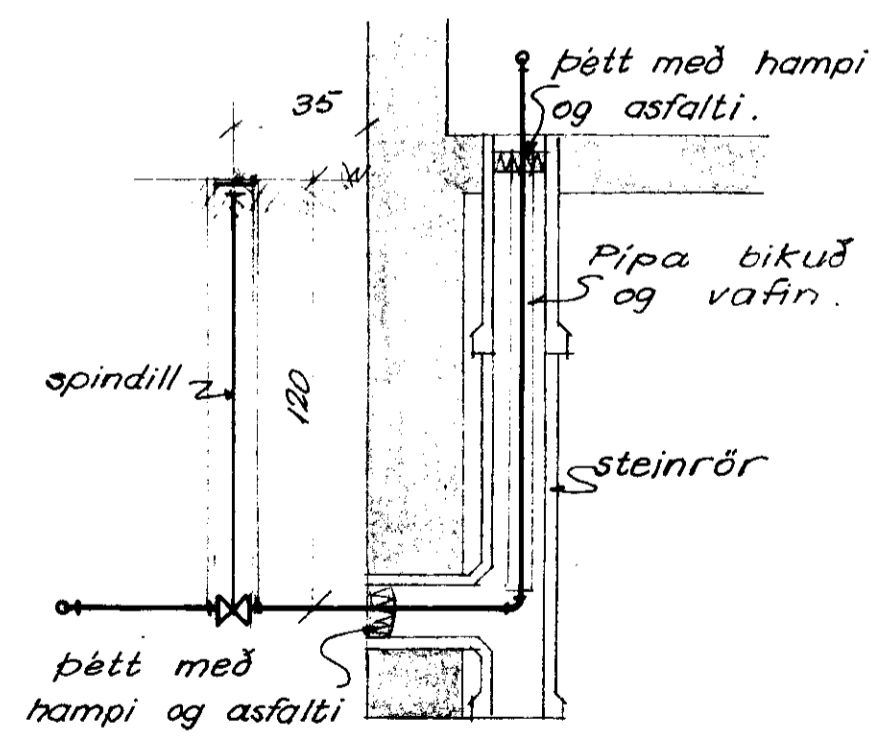
INNTAK 1:20
