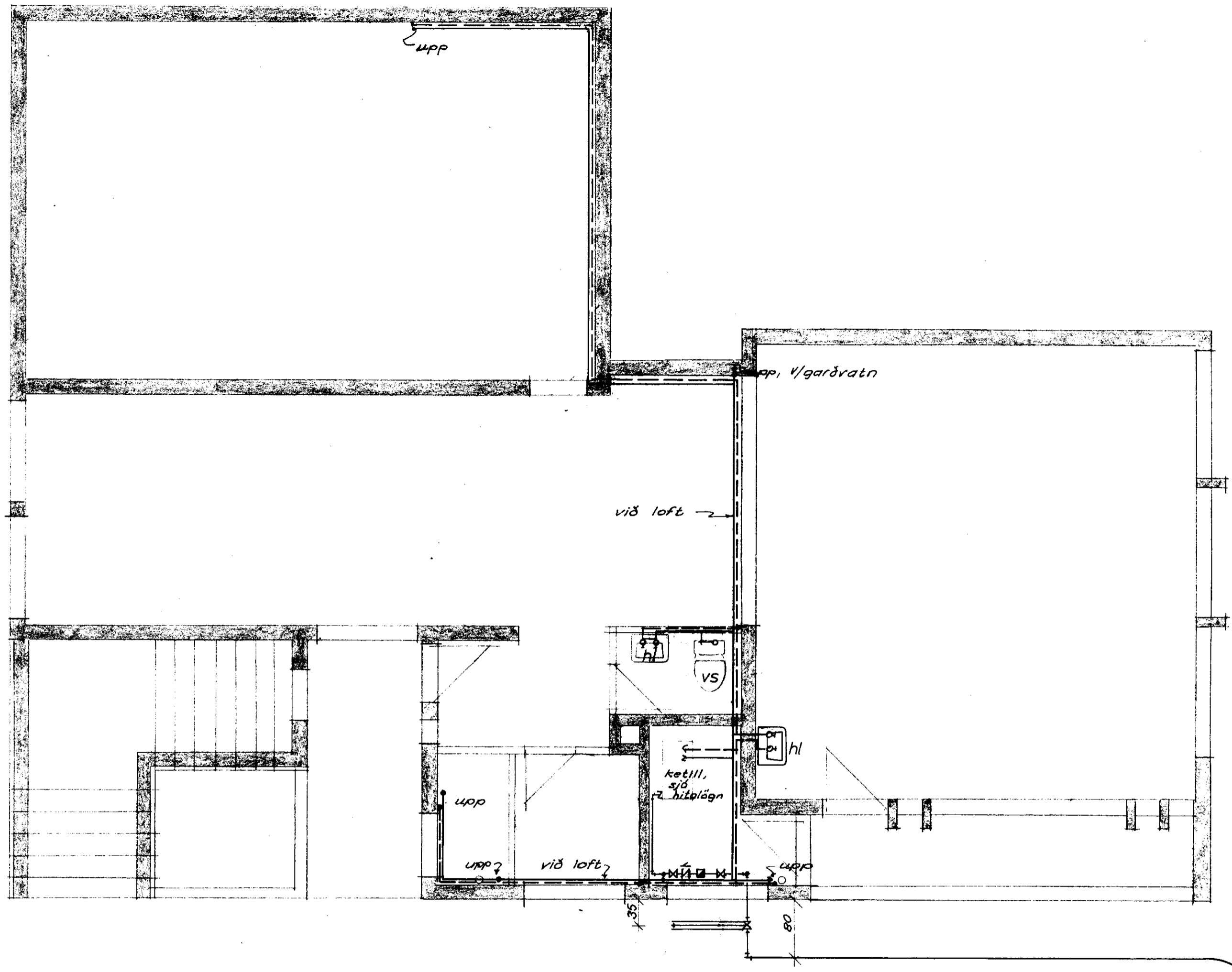
GRUNNMYND KJALLARI 1:50.
