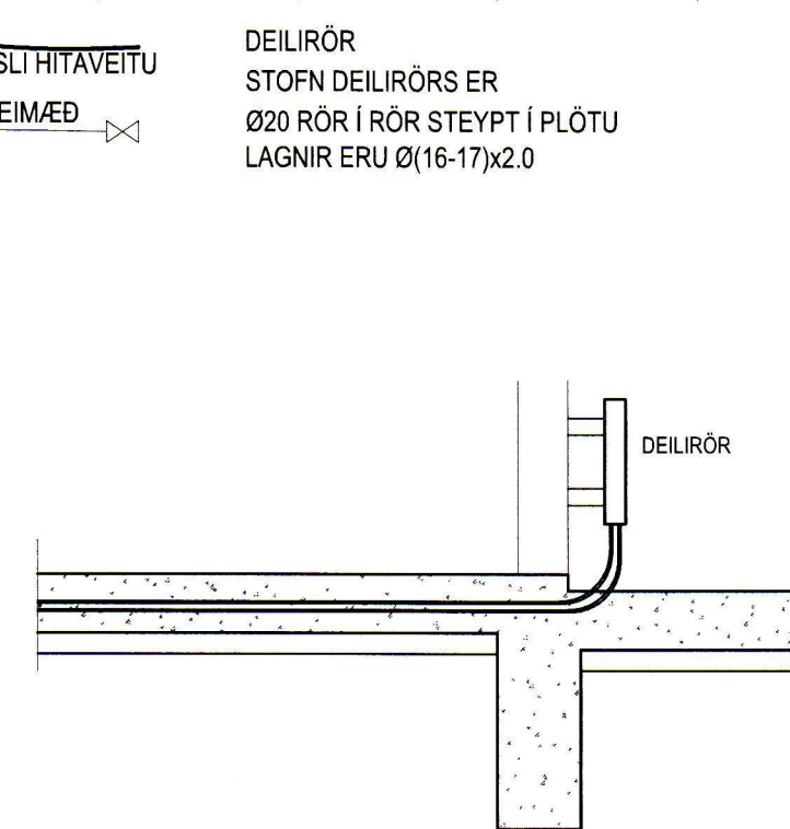
FRÁG. LAGNA Á MÓTUM BÍLSKÚRS OG ÍBÚÐAR MKV: 1:20
