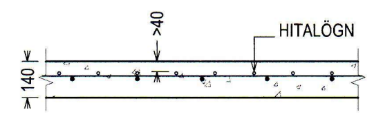
STAÐSETNING HITALAGNA Í BÍLSKÚR MKV: 1:20
