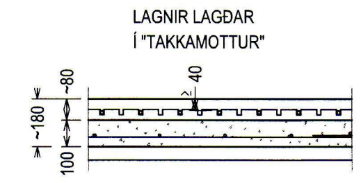
STAÐSETNING HITALAGNA Í ÍBÚÐ MKV: 1:20
