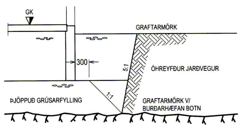
GRUNDUN Mkv. 1:50
