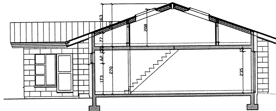
SNID D-D
