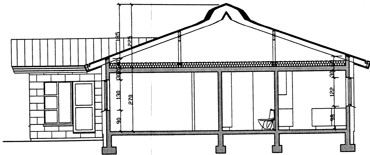
SNID A-A
