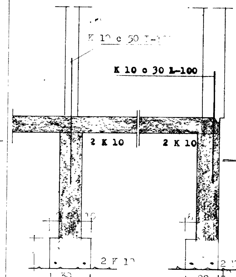
UNDIRSTADA INNVEGGJA SNID - C 1:20
