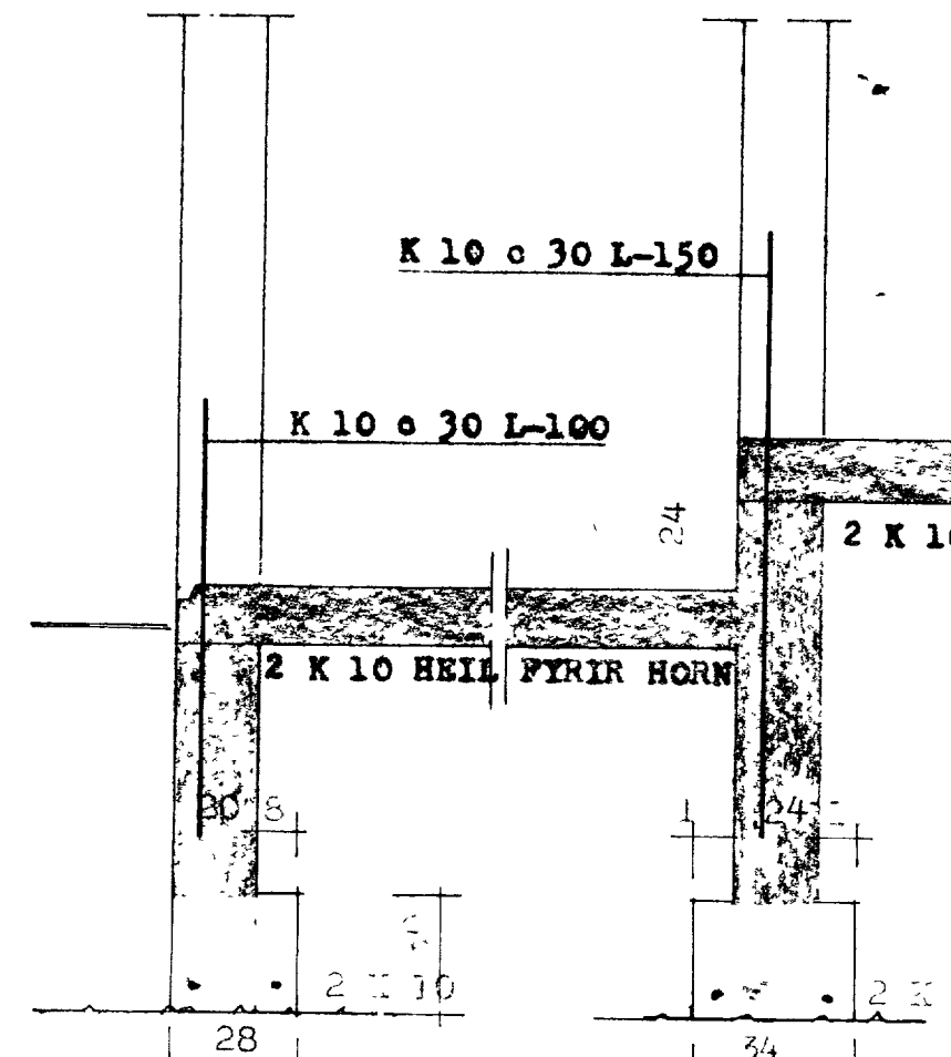
UNDIRSTADA BILSKURS SNID - A 1:20
