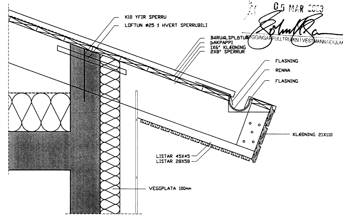
ÞAKKASSI SNID
