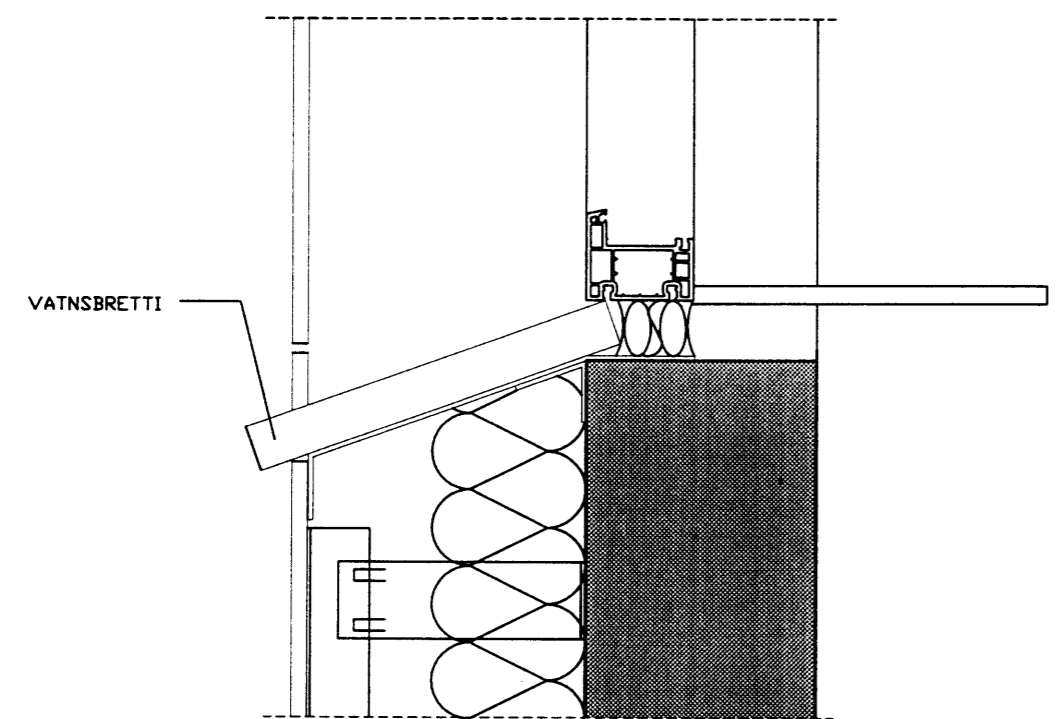
LÓÐRÉTT SNID
