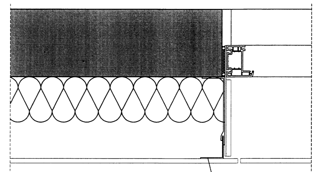
LÁRÉTT SNID
