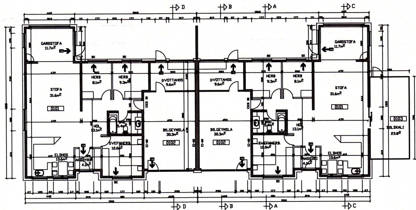
GRUNNMYND
