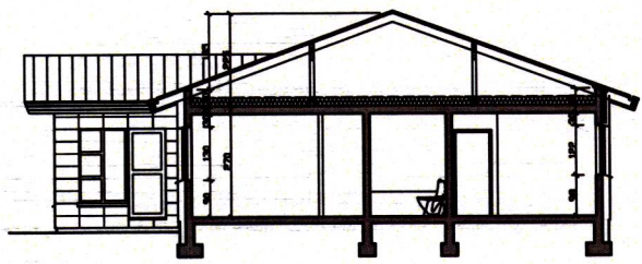
SNID A-A
