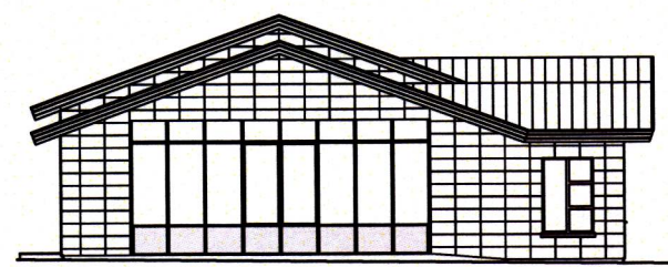
VESTURHLID
