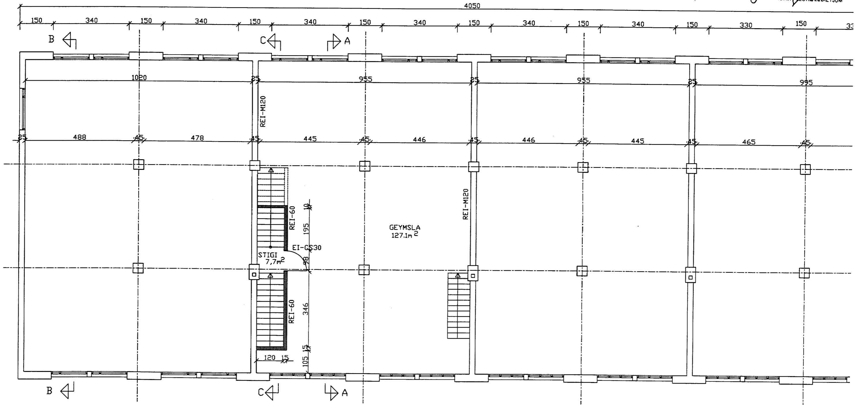
GRUNNMYND 2. HÆÐ
