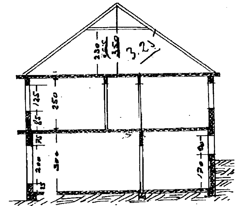
SKURÐUR
