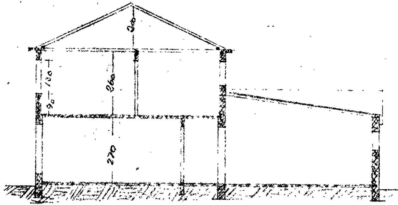
SKURÐUR A-B
