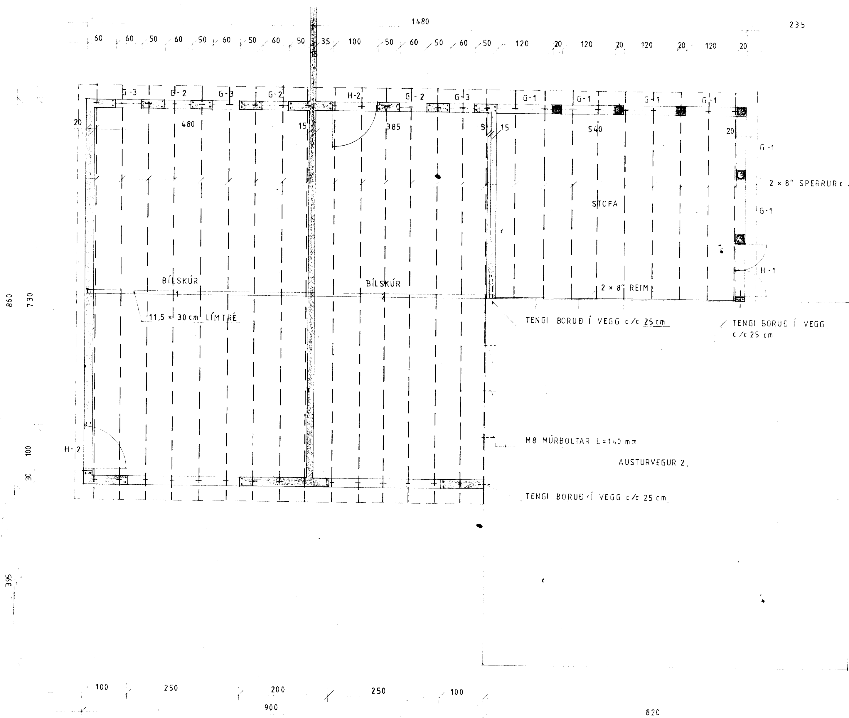
GRUNNMYND 1:50
