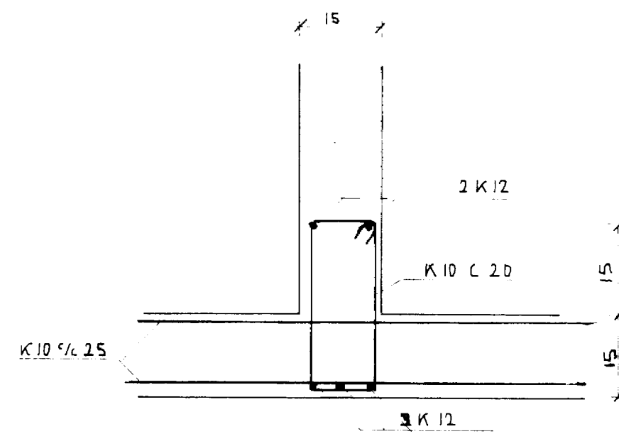
SNID D-D MKV 1:10
