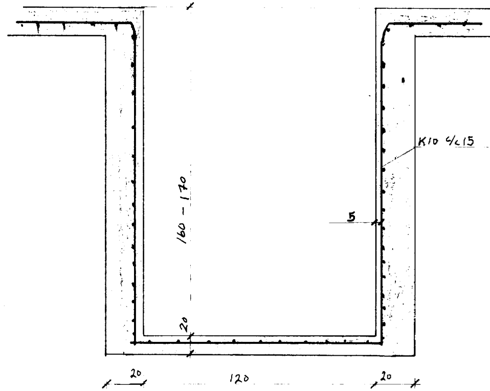
SNID D-D MKV 1:10
