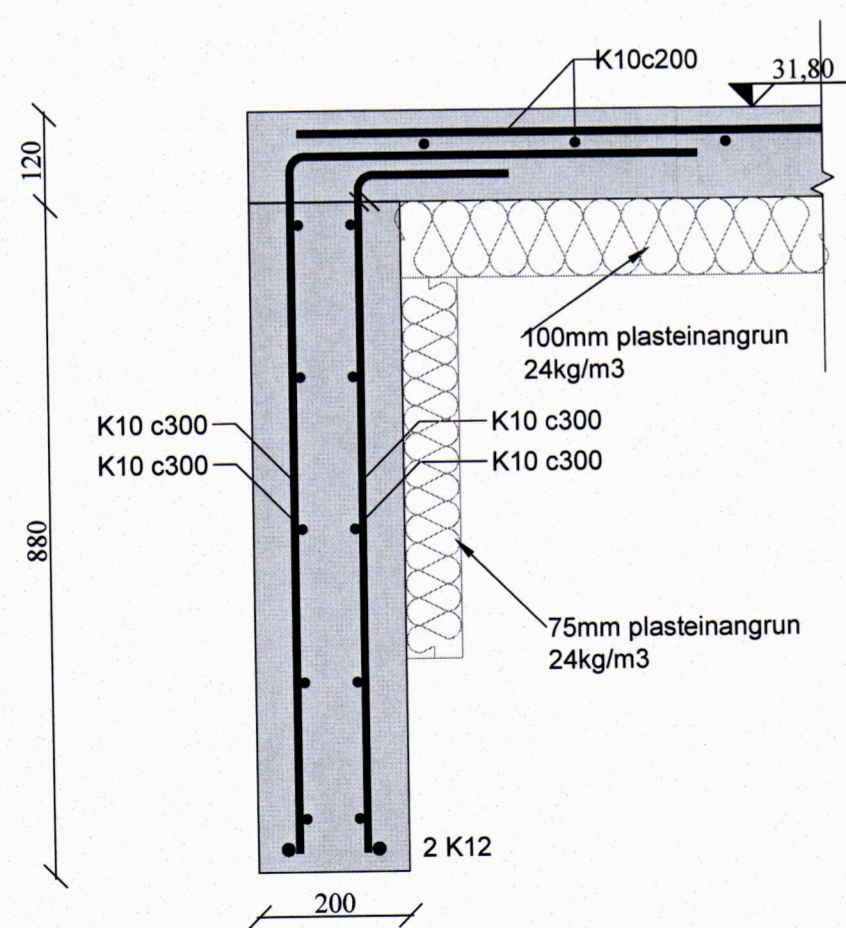
Snið D 1:10
