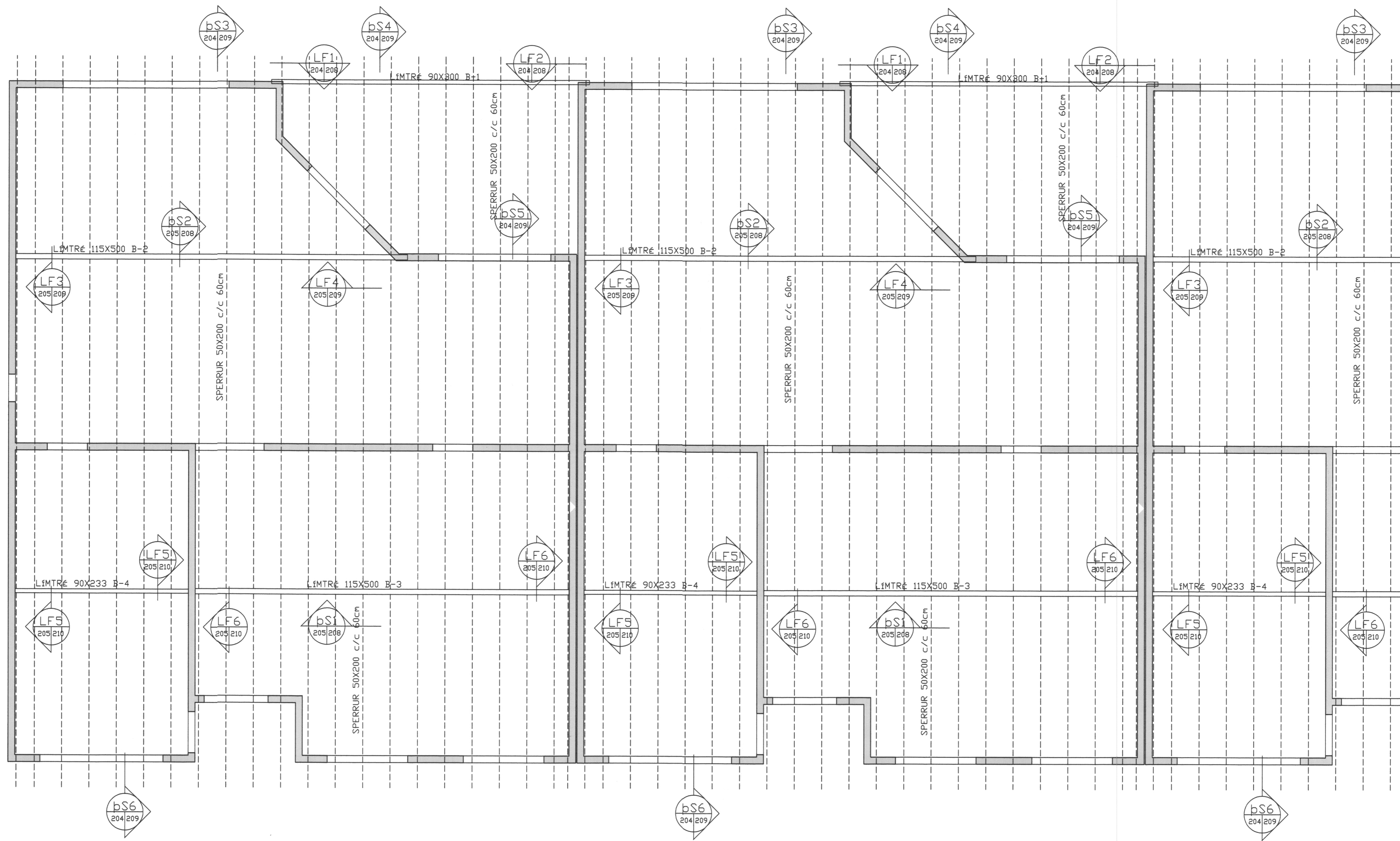
GRUNNMYND SUBURHLUTI
