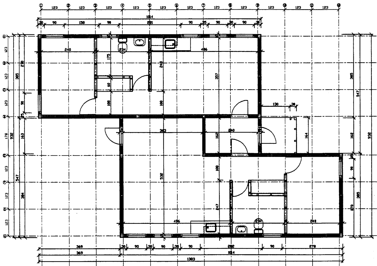
GRUNNMYND
