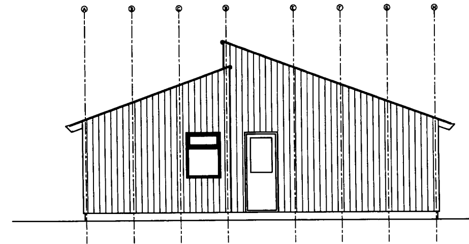
VESTURHLIÐ
