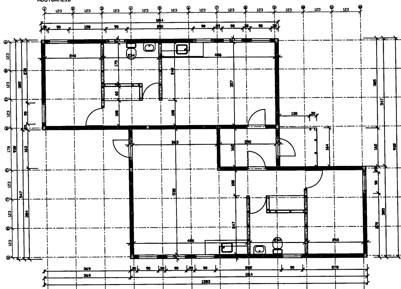
GRUNNMYND
