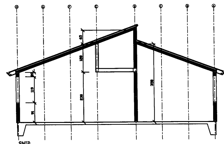
SNIÐ
